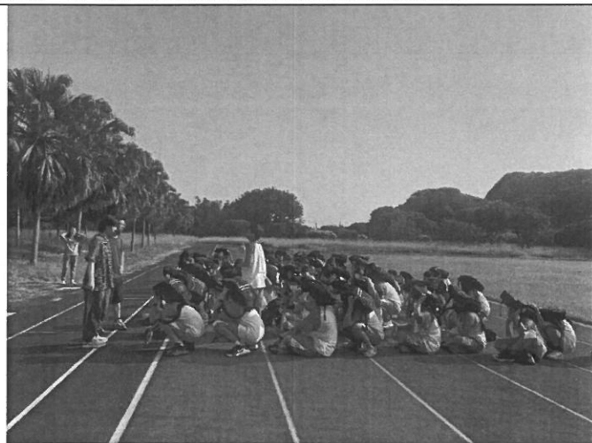
地點：學校操場 時間：112.9.21 說明：學生抵達安全疏散地點，清點班級人數
